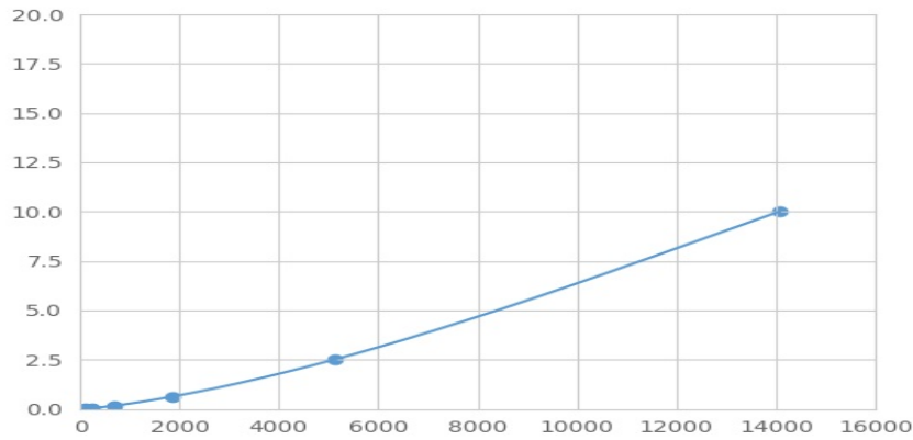
(多胺调节因子1结合蛋白1)检测试剂盒标准曲线
