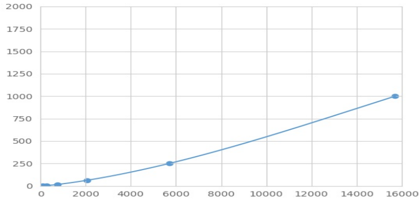
(多聚免疫球蛋白受体)检测试剂盒标准曲线
