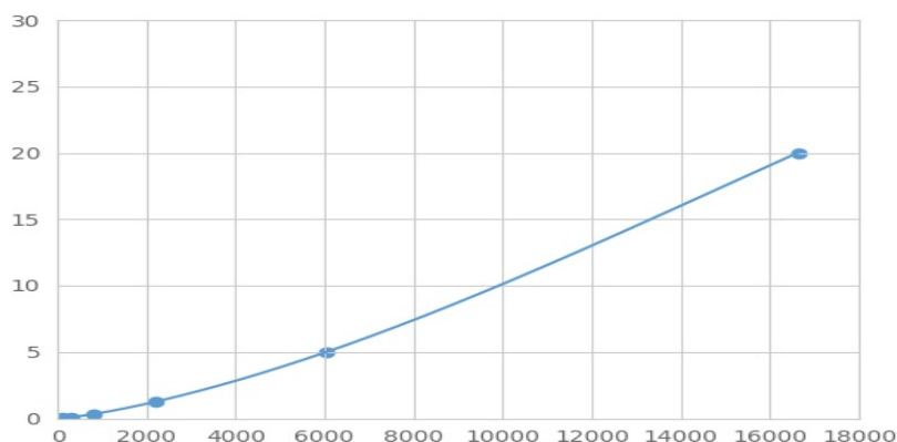
(非受体型蛋白酪氨酸磷酸酶11)检测试剂盒标准曲线
