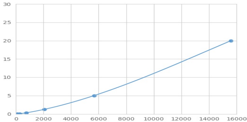
(原钙黏素20)检测试剂盒标准曲线
