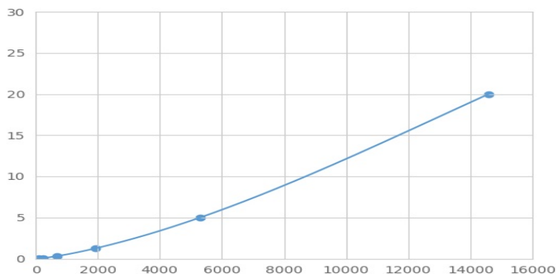
(视黄醇结合蛋白4)检测试剂盒标准曲线
