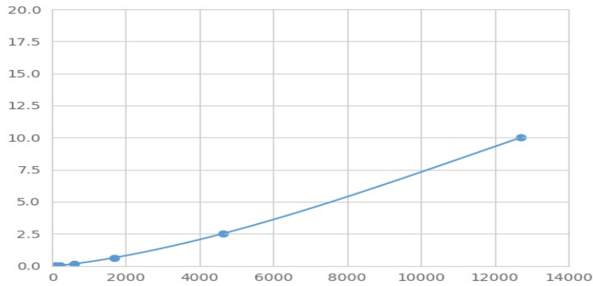
(核糖体蛋白L36A样蛋白)检测试剂盒标准曲线
