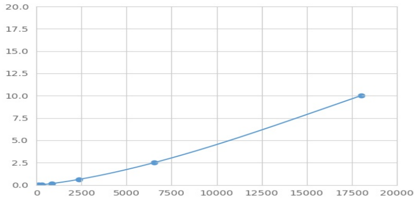
(S-期激酶关联蛋白1)检测试剂盒标准曲线
