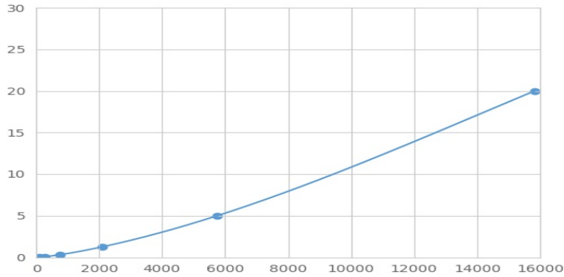
(丝氨酸蛋白酶抑制因子Kazal1型5)检测试剂盒标准曲线
