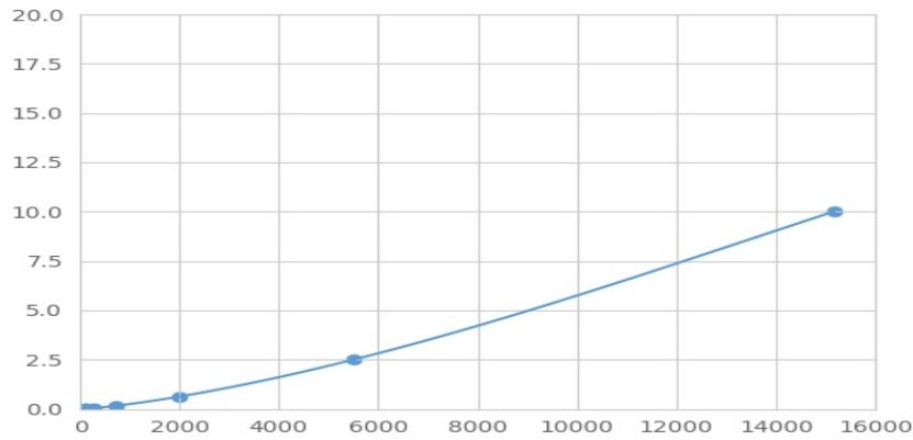
(前列腺六跨膜表皮抗原2)检测试剂盒标准曲线
