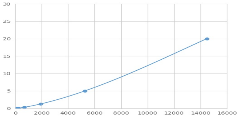
(胞浆磷蛋白2)检测试剂盒标准曲线
