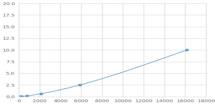
(亚硫酸盐氧化酶)检测试剂盒标准曲线
