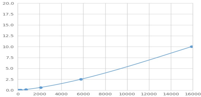
(Syncollin蛋白)检测试剂盒标准曲线
