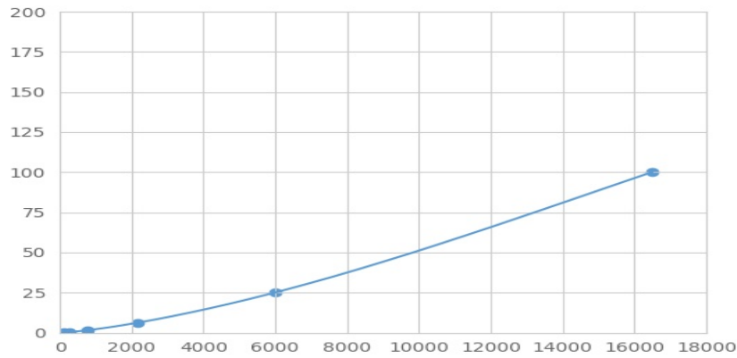
(色氨酸酰tRNA合成酶)检测试剂盒标准曲线
