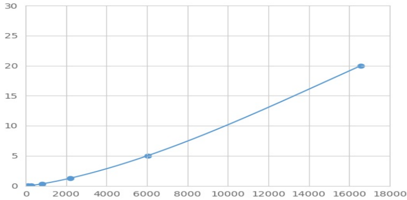
(微管蛋白 \alpha 1A) 检测试剂盒标准曲线
