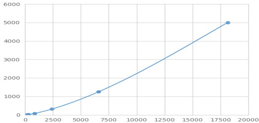
(肿瘤坏死因子 \alpha 诱导蛋白6)检测试剂盒标准曲线
