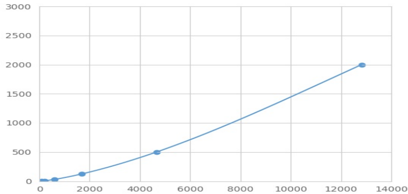
(肿瘤坏死因子受体超家族成员12A)检测试剂盒标准曲线
