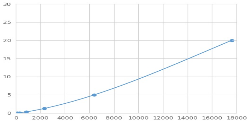
(肿瘤蛋白p53结合蛋白1)检测试剂盒标准曲线
