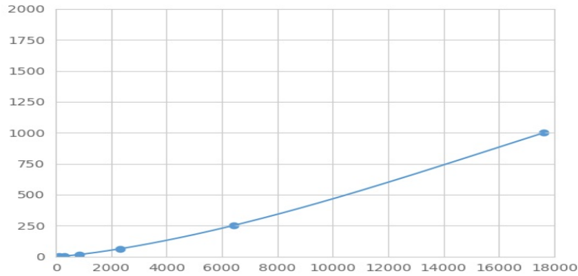
(血管内皮生长因子183)检测试剂盒标准曲线
