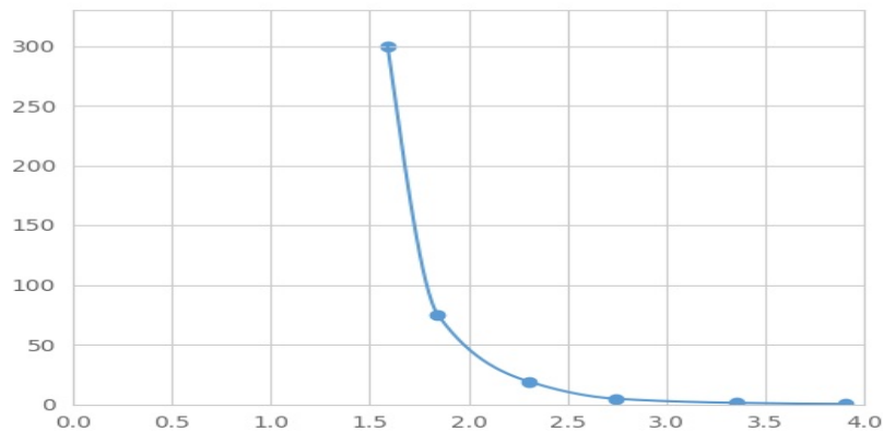
(维生素B1)检测试剂盒标准曲线
