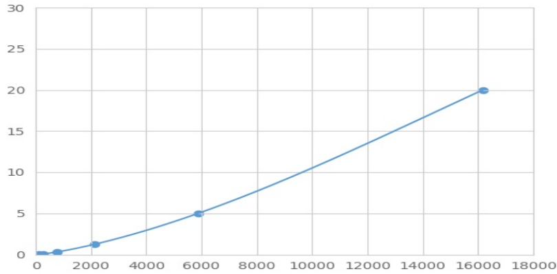
(WNT1诱导信号通道蛋白2)检测试剂盒标准曲线
