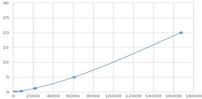
(酶原蛋白16同源物B)检测试剂盒标准曲线
