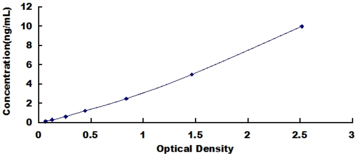
人酸性神经鞘磷脂酶(ASM)检测试剂盒标准曲线
