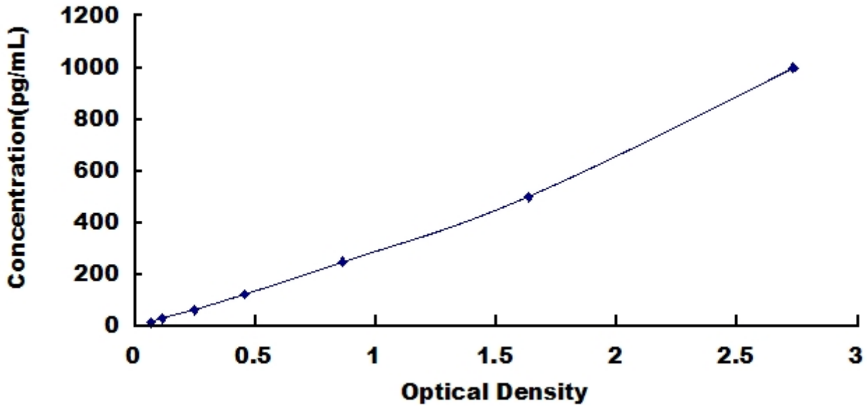
人白介素 21 (IL21) 检测试剂盒标准曲线
