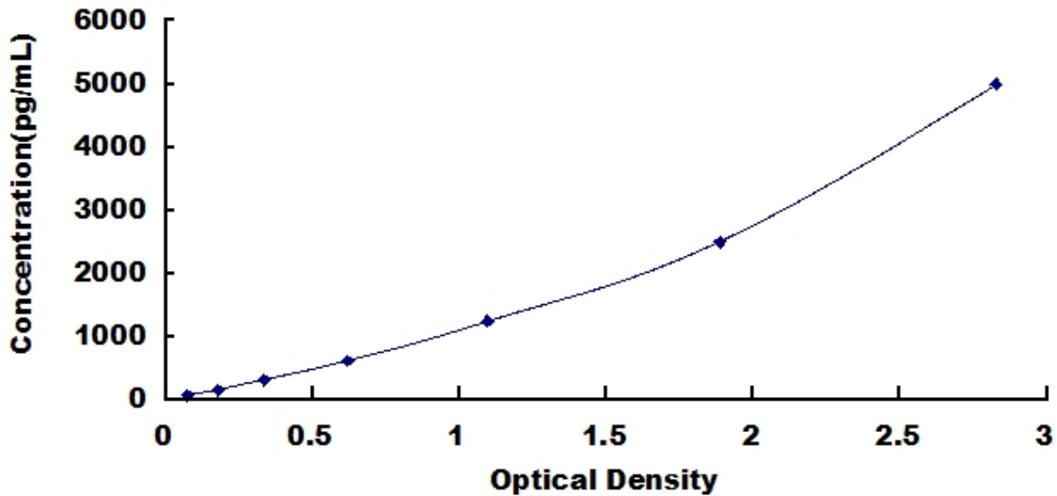
小鼠调节激活正常 T-细胞表达分泌因子(RANTES)检测试剂盒标准曲线
